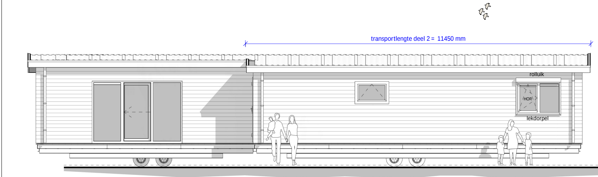
VOORGEVEL
