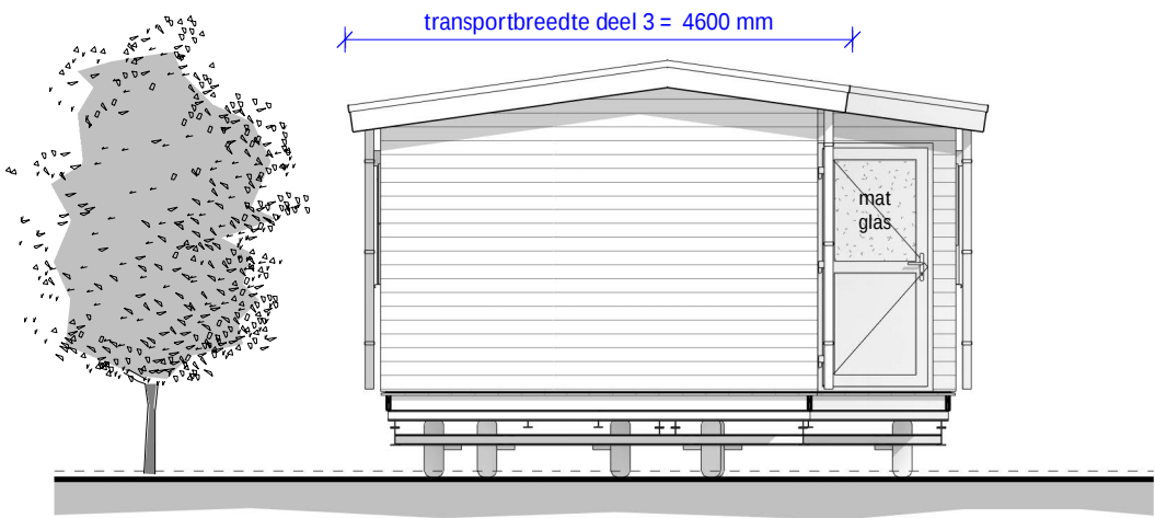
LINKERZIJGEVEL
