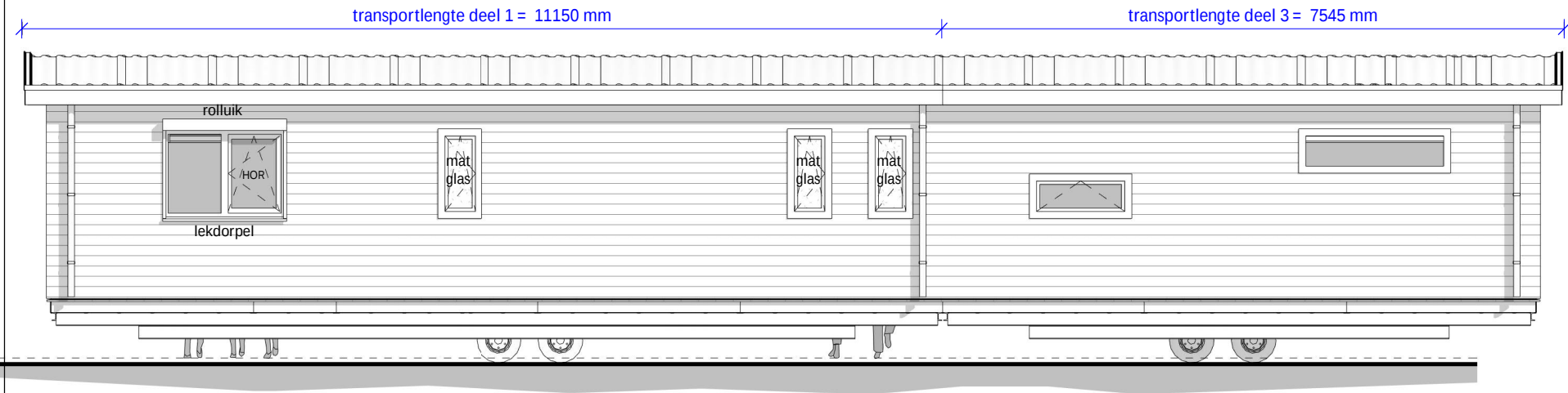
ACHTERGEVEL
