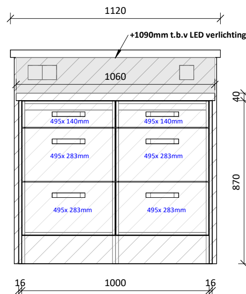
eiland aanzicht 1
