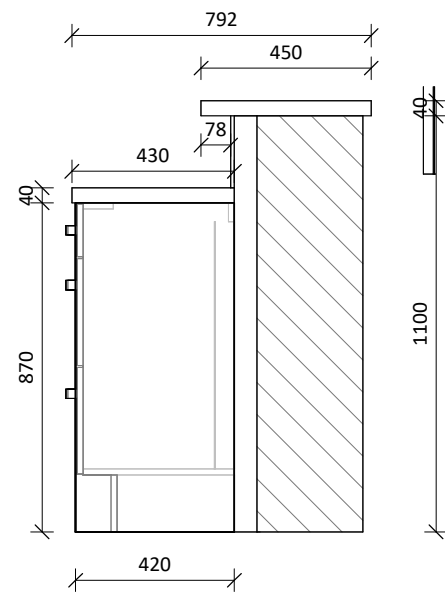
eiland aanzicht 2
